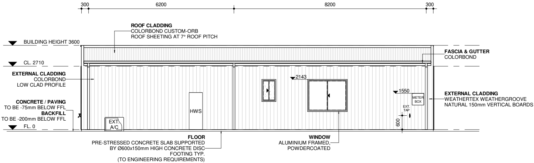
E1 E1 ELEVATION A103 1 : 100
