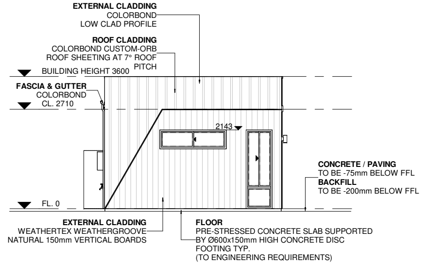
E2 E2 ELEVATION A103 1 : 100
