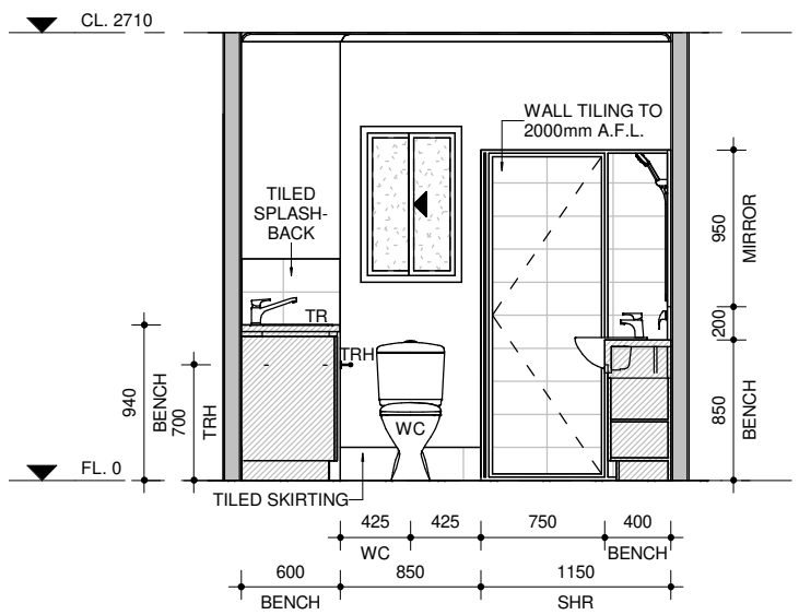
B2 B2 BATH A106 1 : 50
