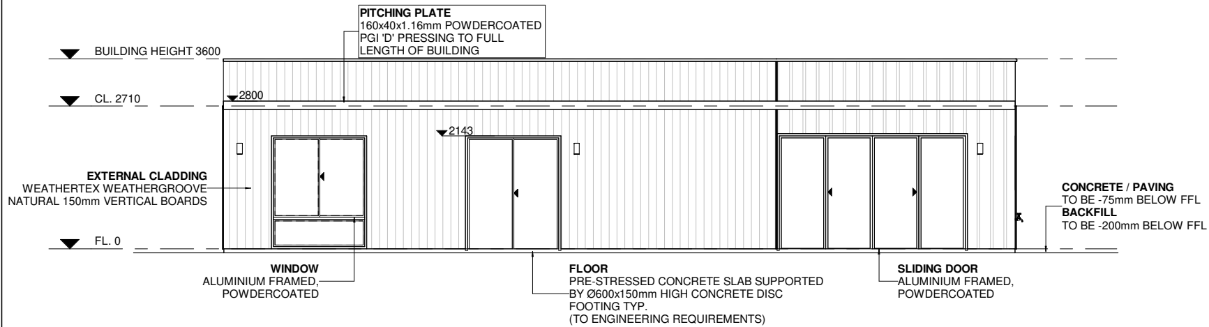
E3 E3 ELEVATION A103 1 : 100
