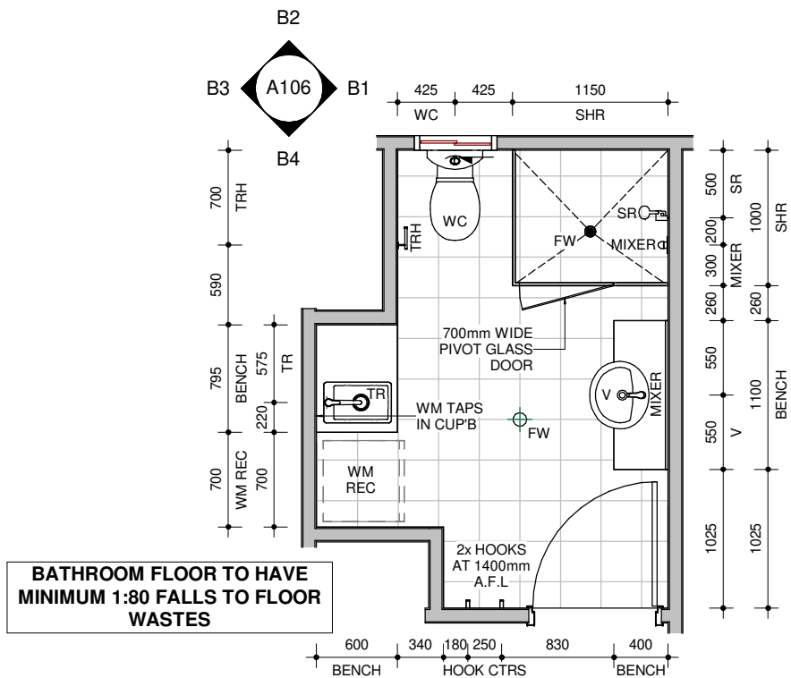
B BATH LAYOUT A106 1 : 50
