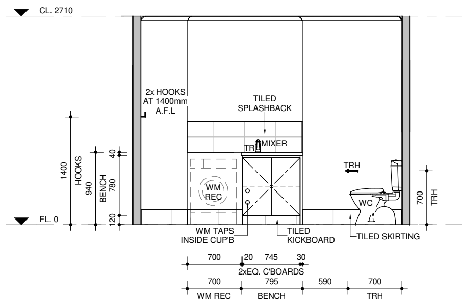
B3 B3 BATH A106 1 : 50
