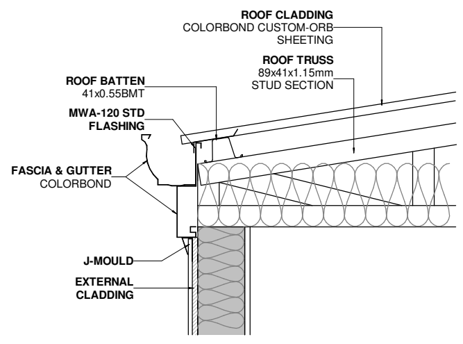
D1 GUTTER DETAIL A107 1 : 10
