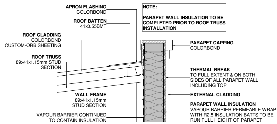
D2 PARAPET DETAIL A107 1 : 10
